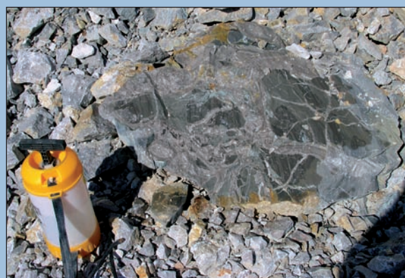
Foto 2. Brekcie s ostrohrannými úlomky páskovaných a laminovaných kotýzských vápenců a téměř zaoblenými úlomky světle šedých kalcilitů tmelená laminovanými freatickými tmely a s vnitřními sedimenty (etáž 360; foto J. Hladil, 14.10. 2003).
